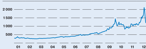
Цена на природный газ «на месяц вперед», торговая площадка TTF, 2021 г., долл./тыс. м 3
