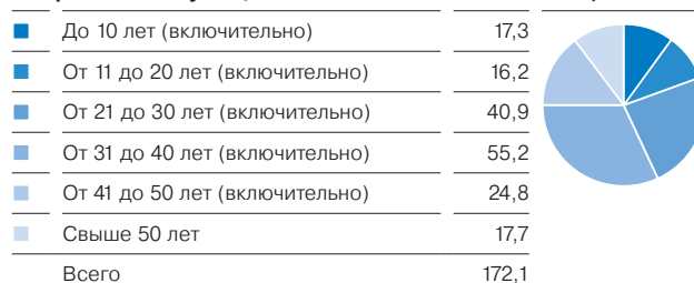
Распределение протяженности магистральных газопроводов газотранспортных обществ Группы на территории России по срокам эксплуатации по состоянию на 31.12.2017 г., тыс. км
